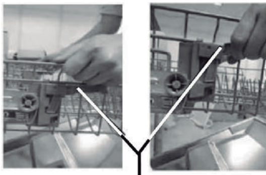
Mecanismo de ajuste da altura do cesto superior
